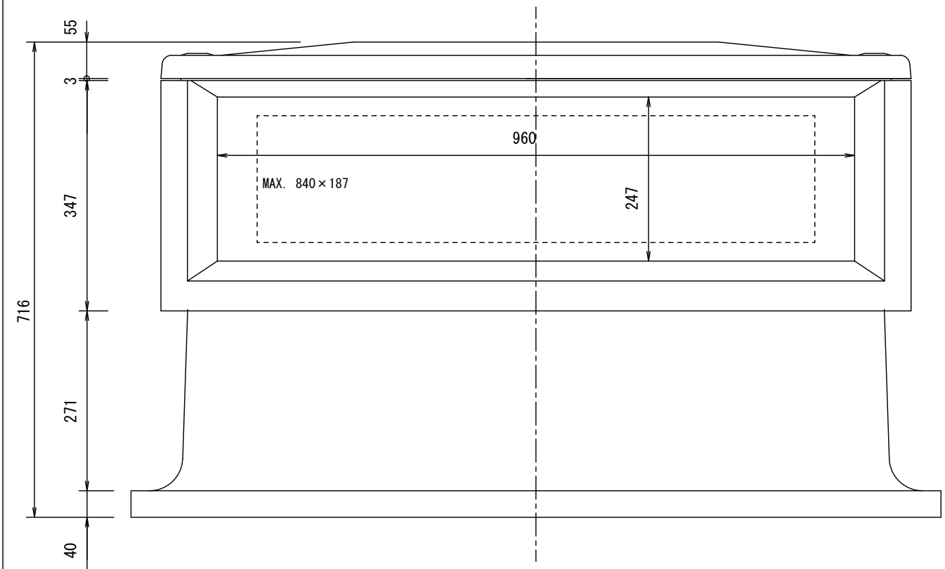
立面図
