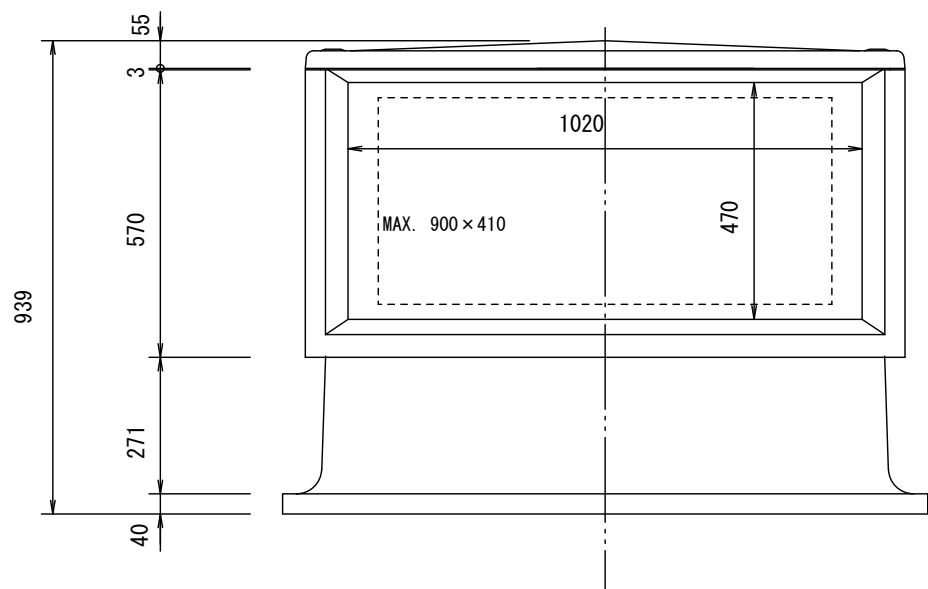
立面図
