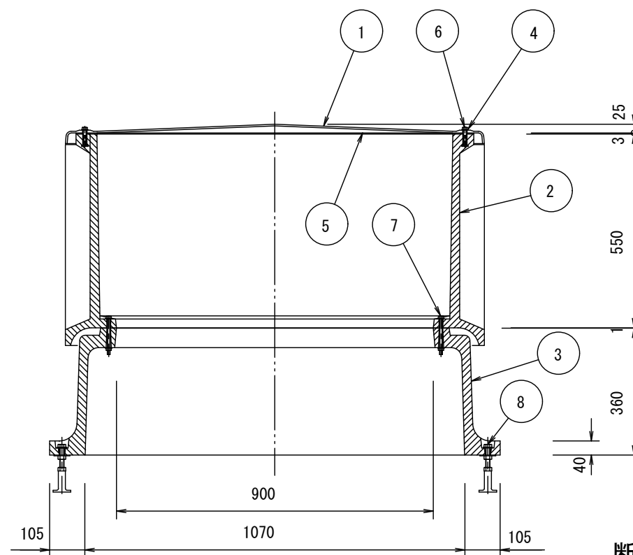
断面図
