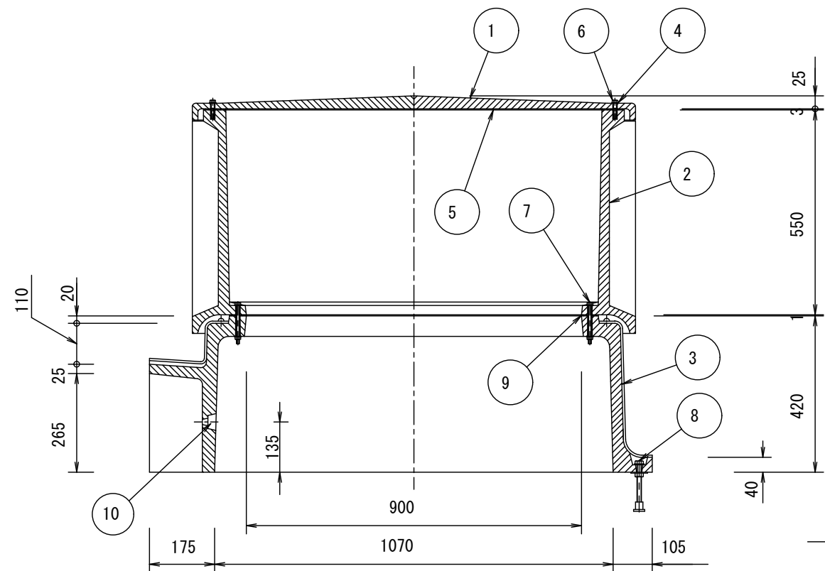
断面図
