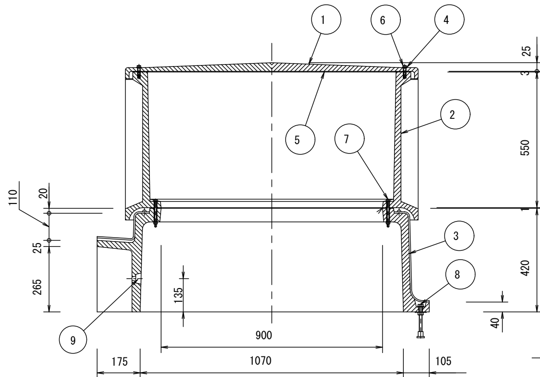
断面図
