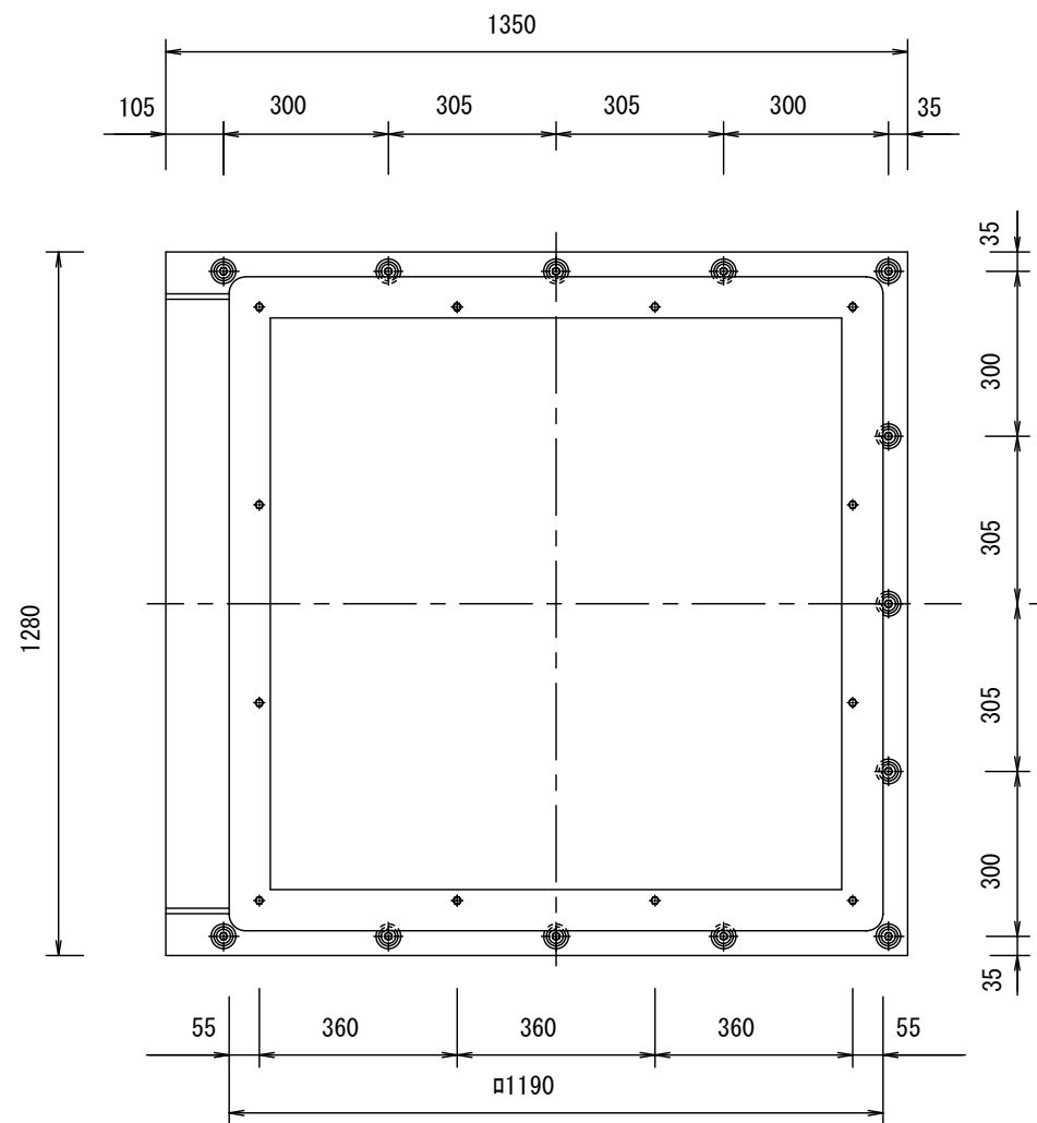
平面図
